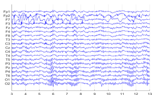
Denoised EEG
