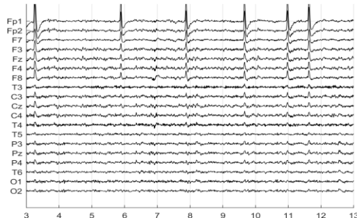
Raw EEG
