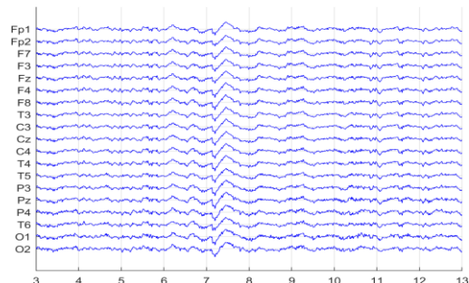
Denoised EEG
