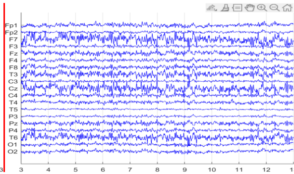
Denoised EEG
