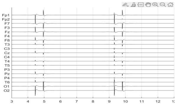
Raw EEG
