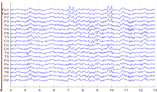
Denoised EEG
