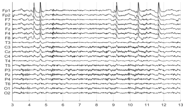
Raw EEG
