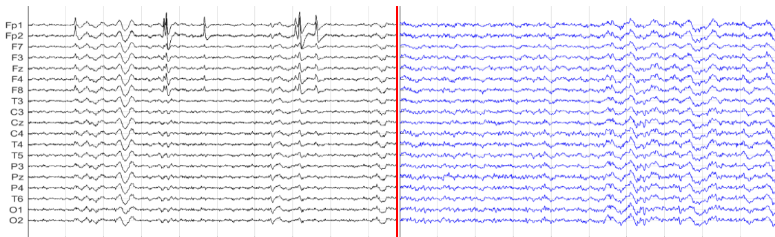
Raw EEG
