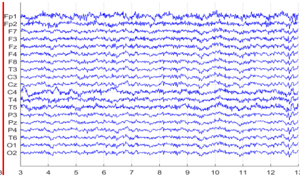
Denoised EEG
